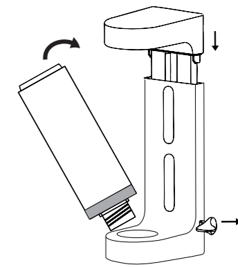
Výměna patrony Cartridge exchange Ersetzung der Patrone Changement de recharge
